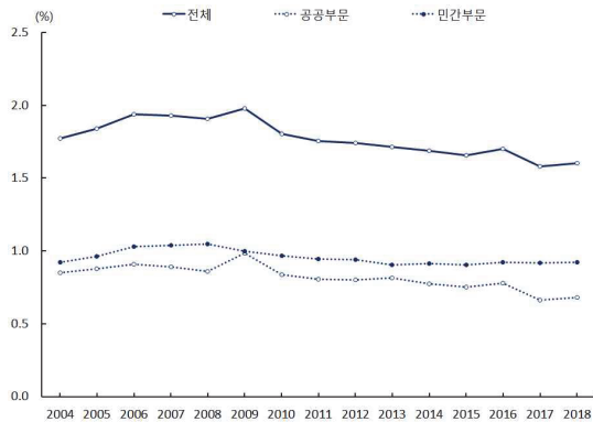
그래프 GDP 대비 환경보호지출 비율, 2004-2018
