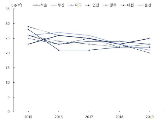
그래프 7대 도시 미세먼지(PM2.5) 농도, 2015-2019
