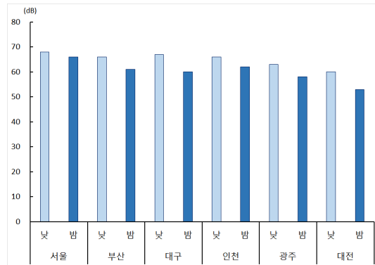
그래프 주요 도시 도로변 주거지역 소음도, 2000-2018
