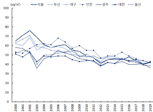
통계표 7대 도시 미세먼지(PM10) 농도, 2000-2019
